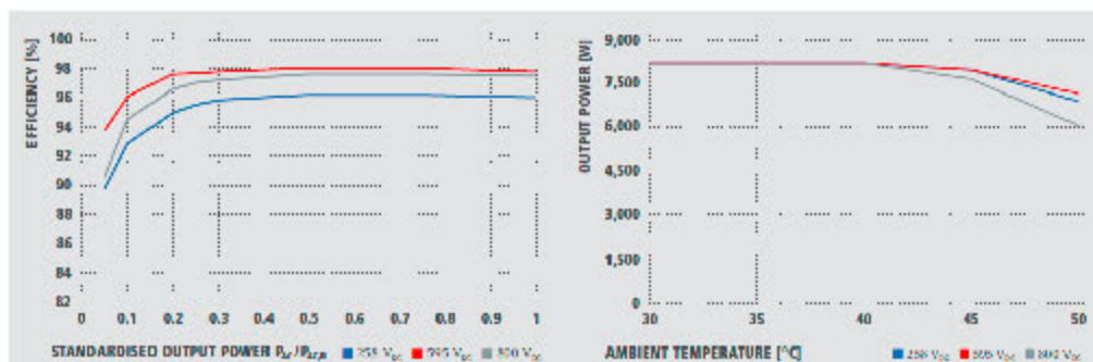
32. ábra Inverterek hatásfok görbéi és hőmérsékletfüggése
