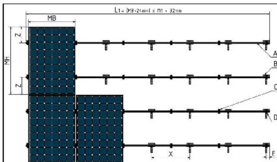
34. ábra Napelemek rögzítése az alumínium síneken
